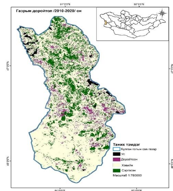
Зураг 7. Газрын доройтол (2010-2020)
