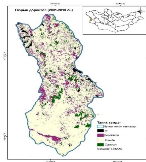
Зураг 6. Газрын доройтол (2001-2010)
