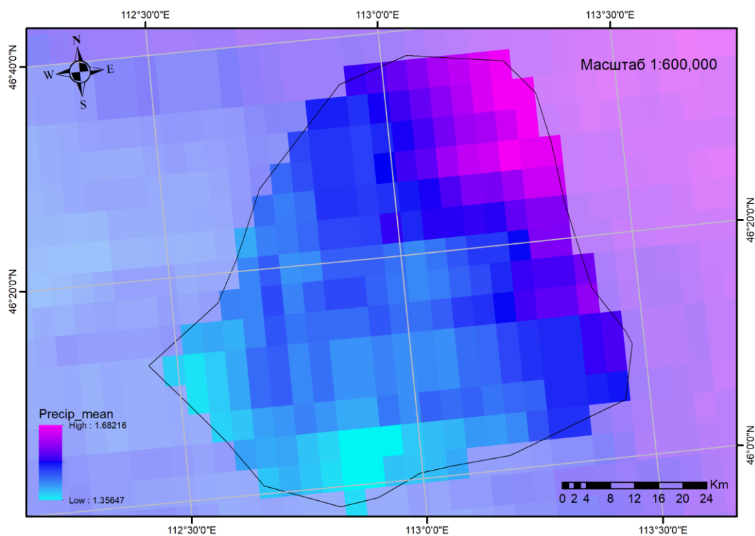
Зураг 10. Хур тунадасны дундаж (2000-2024)
