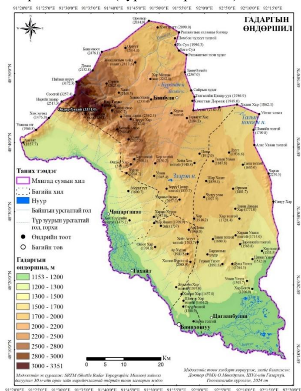
Зураг 4. Гадаргын өндөршил
