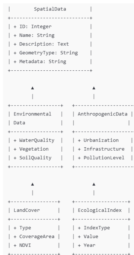
Зураг 1. UML дээрх үндсэн диаграммын загвар
