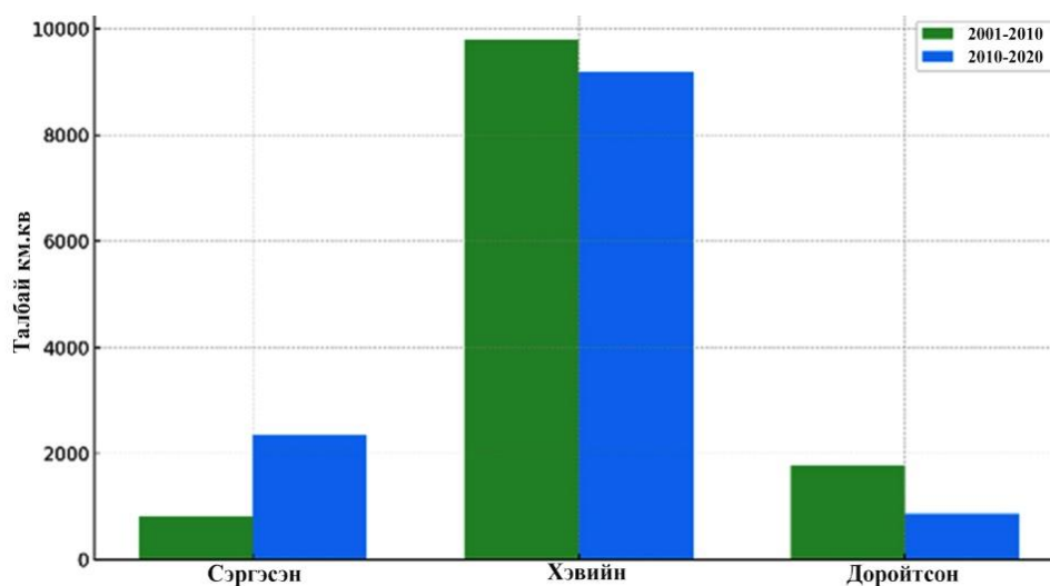
Зураг 5. Газрын доройтлын өөрчлөлт
