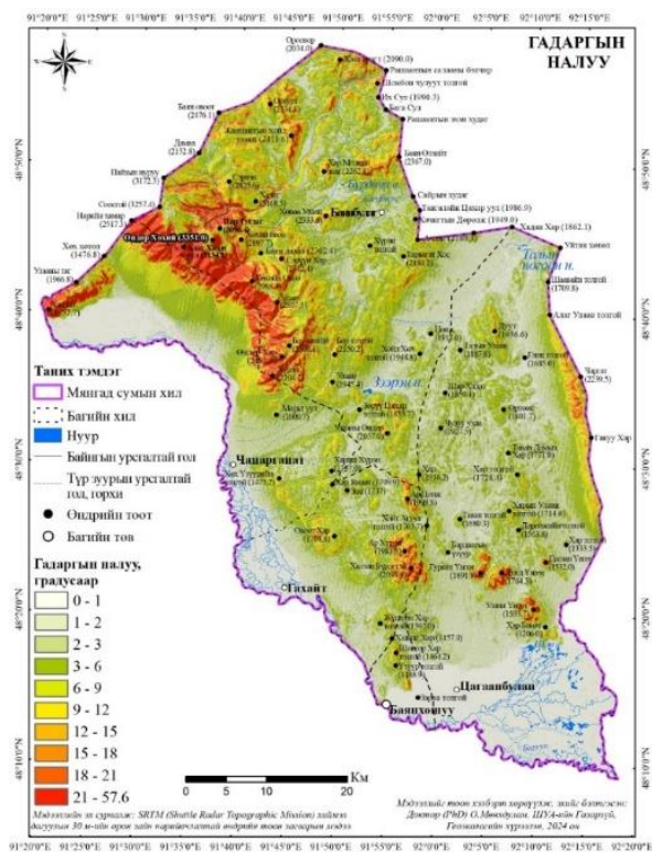
Зураг 5. Гадаргын налуу
