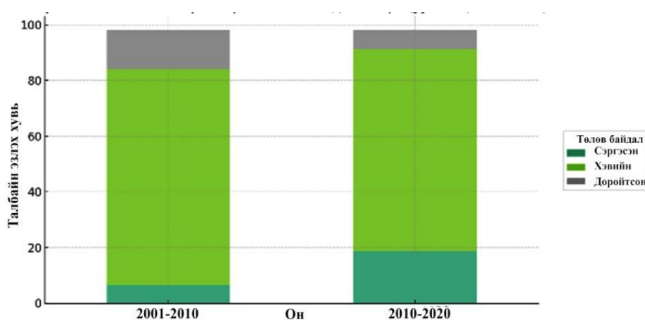
Зураг 4. Газрын төлөв байдлын харьцуулалт
