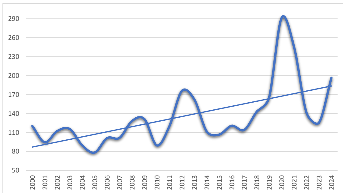
Зураг 9. 2000-2024 оны хур тунадасны өөрчлөлт
